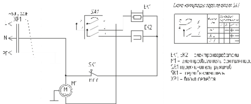
рис. 3 Схема электрическая.
