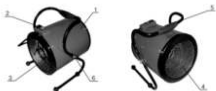
рис. 1 Тепловентилятор
